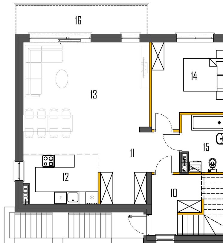
RZUT PIĘTRA
