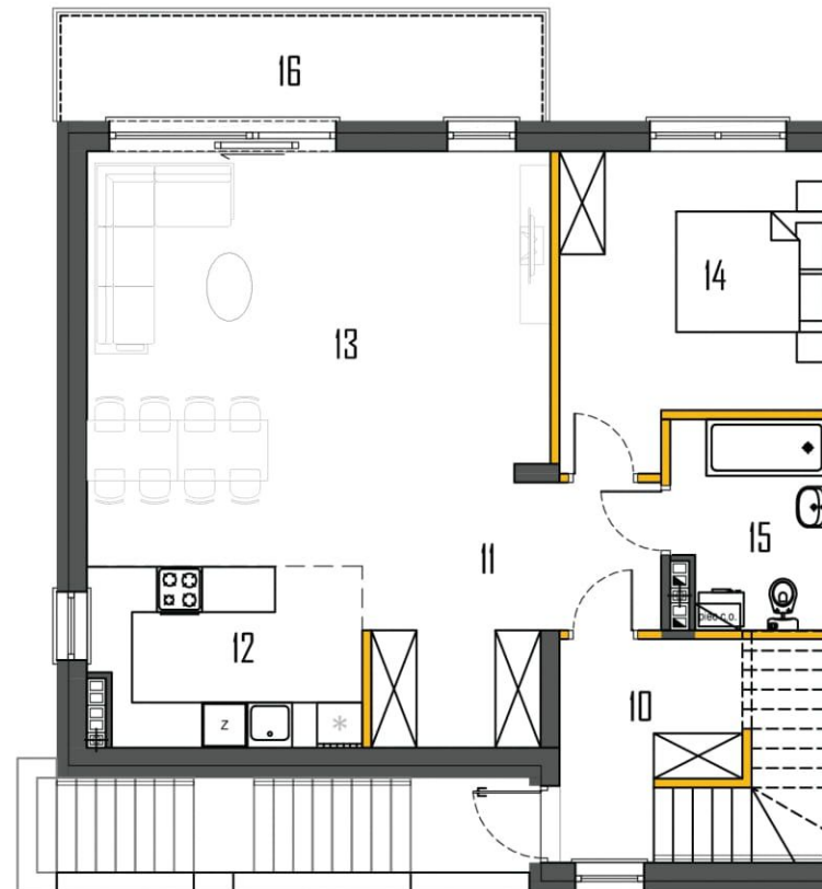
RZUT PIĘTRA
